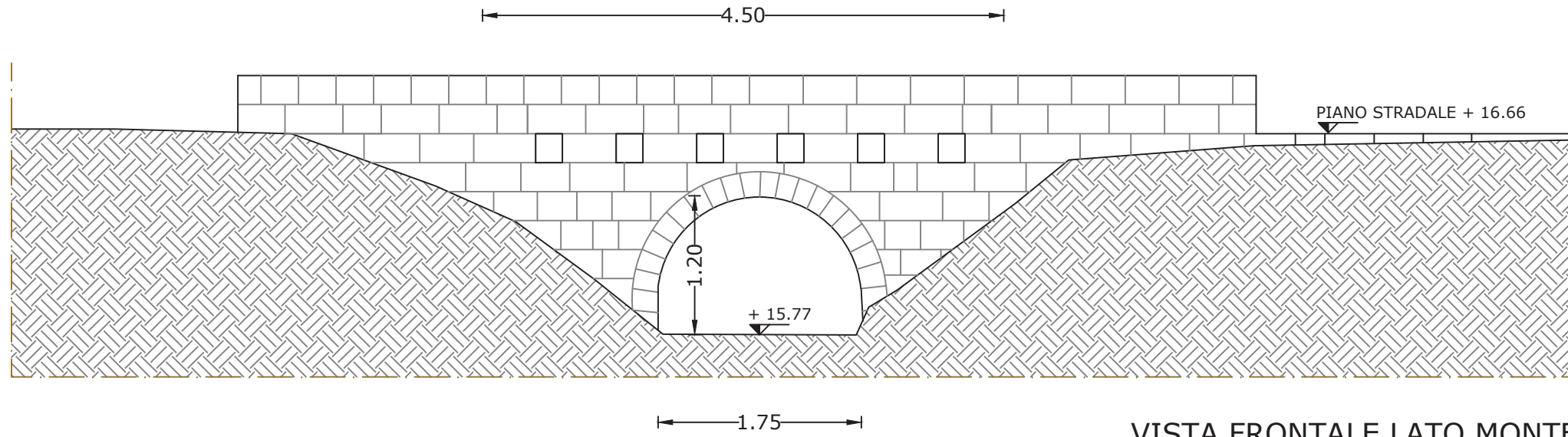
VISTA FRONTALE LATO MONTE scala 1.200
