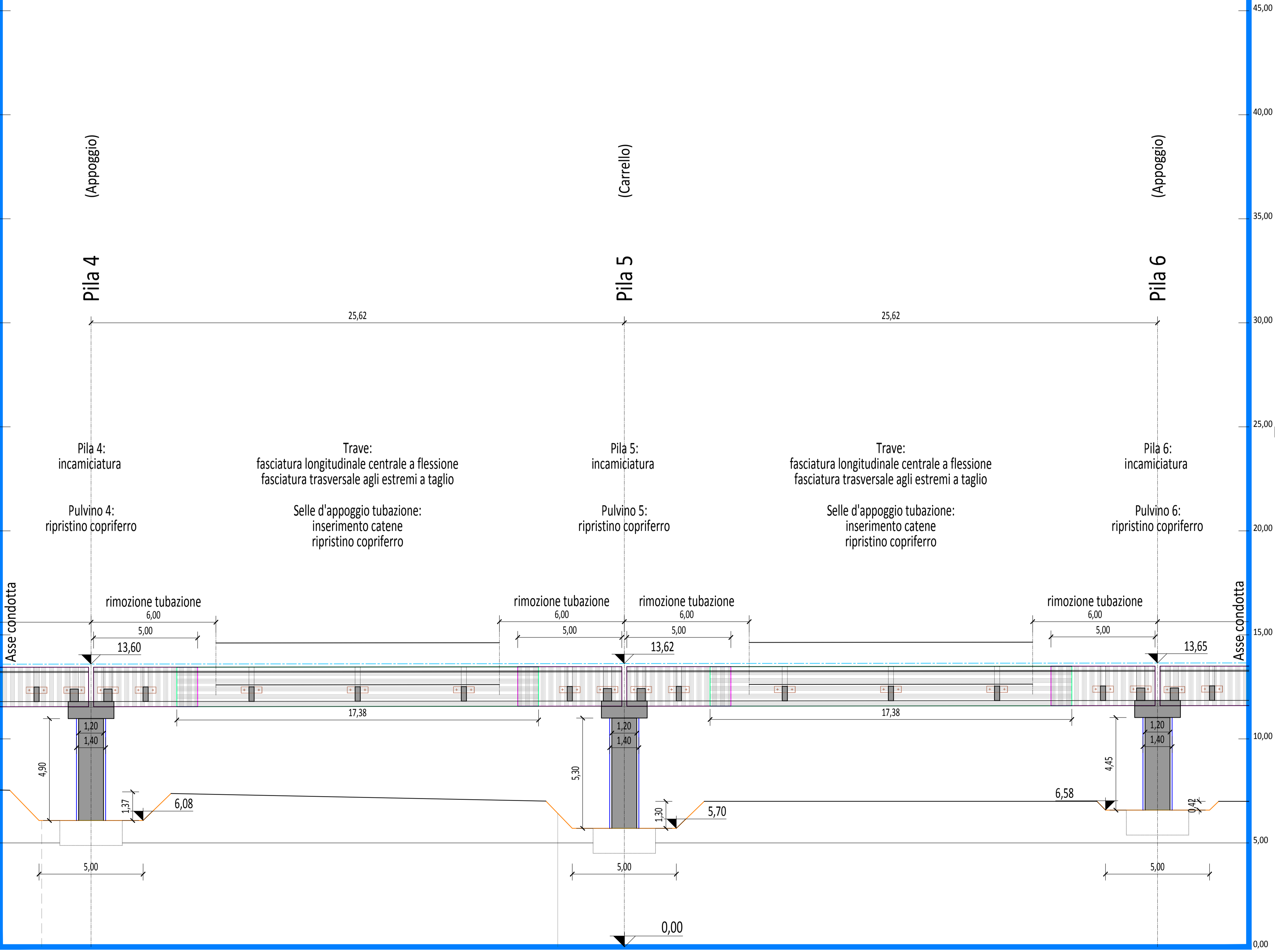
Profilo longitudinale dalla Pila 4 alla Pila 6
